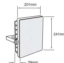
LQ-LED/004/65 LUZ DE DÍA ● 6 500 K
