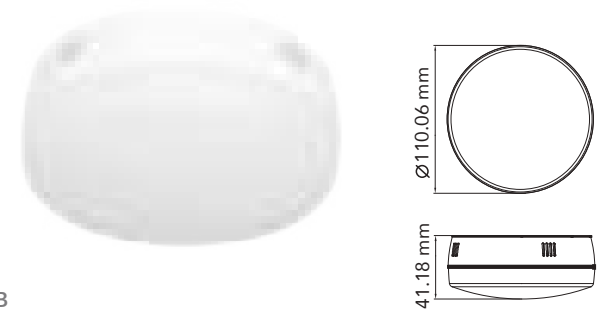
NUEVO C-DOMUS II 09PTLLED4031MV40B LUZ BLANCA NEUTRA ○ 4 000 K
