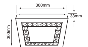
15DPTLLEDC006V40B Lúmenes: 1 600 lm Volts: 127 V ~ Atenuable: Si
