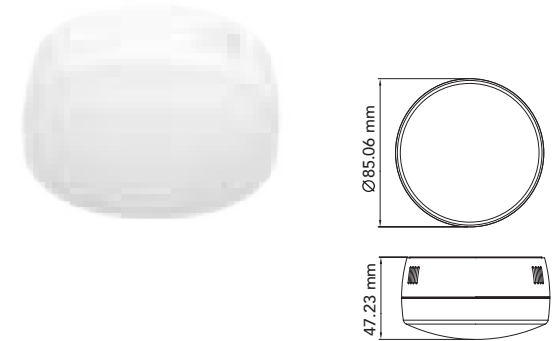
NUEVO C-DOMUS I 7PTLLED4030MV40B LUZ BLANCA NEUTRA ○ 4 000 K
